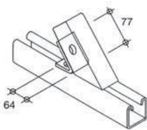
1186 - 45°
